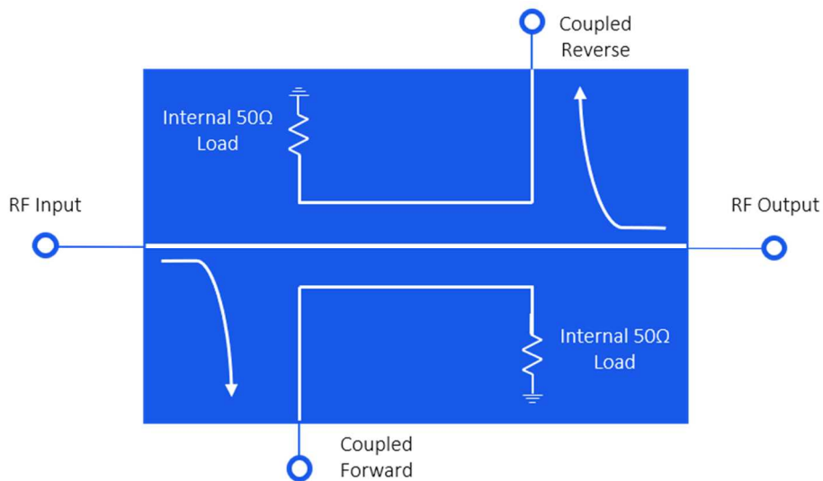
(図 4. デュアル方向性結合器)
