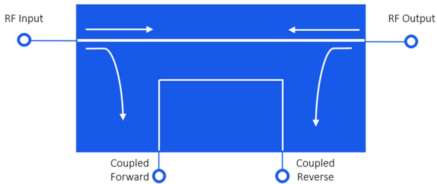
(図 3. 双方向性結合器)
