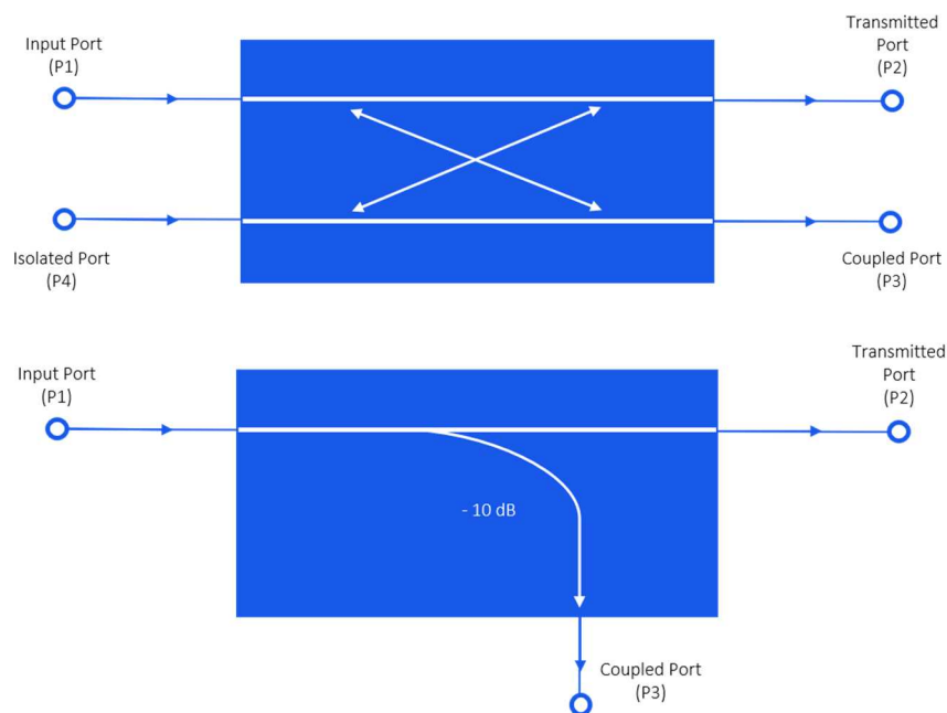
(図1：方向性結合器の基本的構成)
